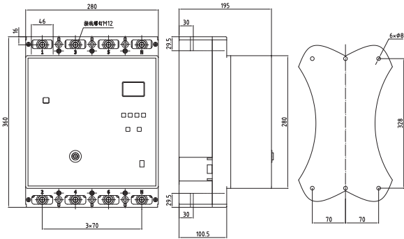
6.4 HUM2DL-800/800A 外形及安装尺寸
