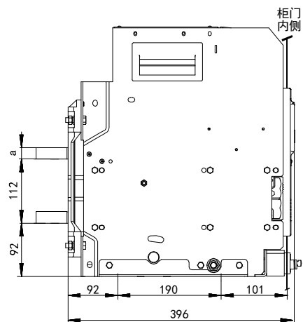
水平接线尺寸
