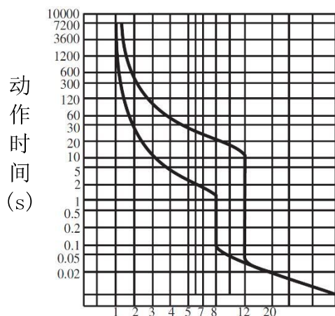
图 7 HYM3-250 动作特性曲线
