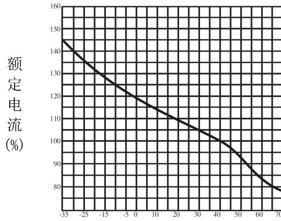
图 10 HYM3-400 温度补偿曲线
