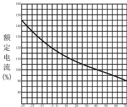
图 6 HYM3-160 温度补偿曲线
