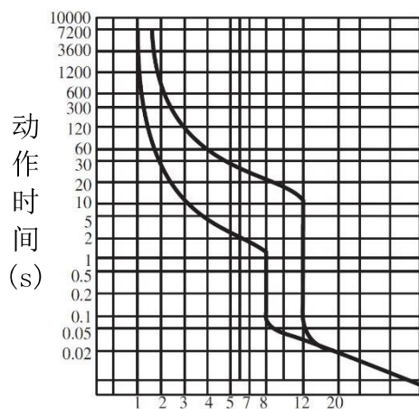
图 5 HYM3-160 动作特性曲线
