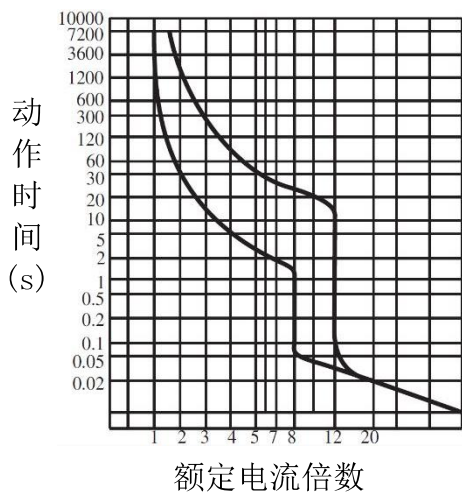
图 3 HYM3-125 动作特性曲线
