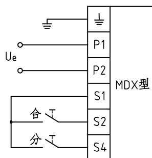
图 17 MDX 型电动操作机构的接线图
