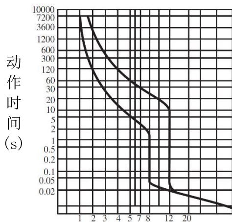
图 9 HYM3-400 动作特性曲线
