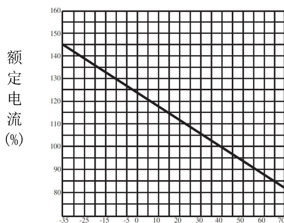
图 8 HYM3-250 温度补偿曲线
